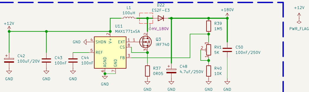
MAX1771 HV Nixie PSU
